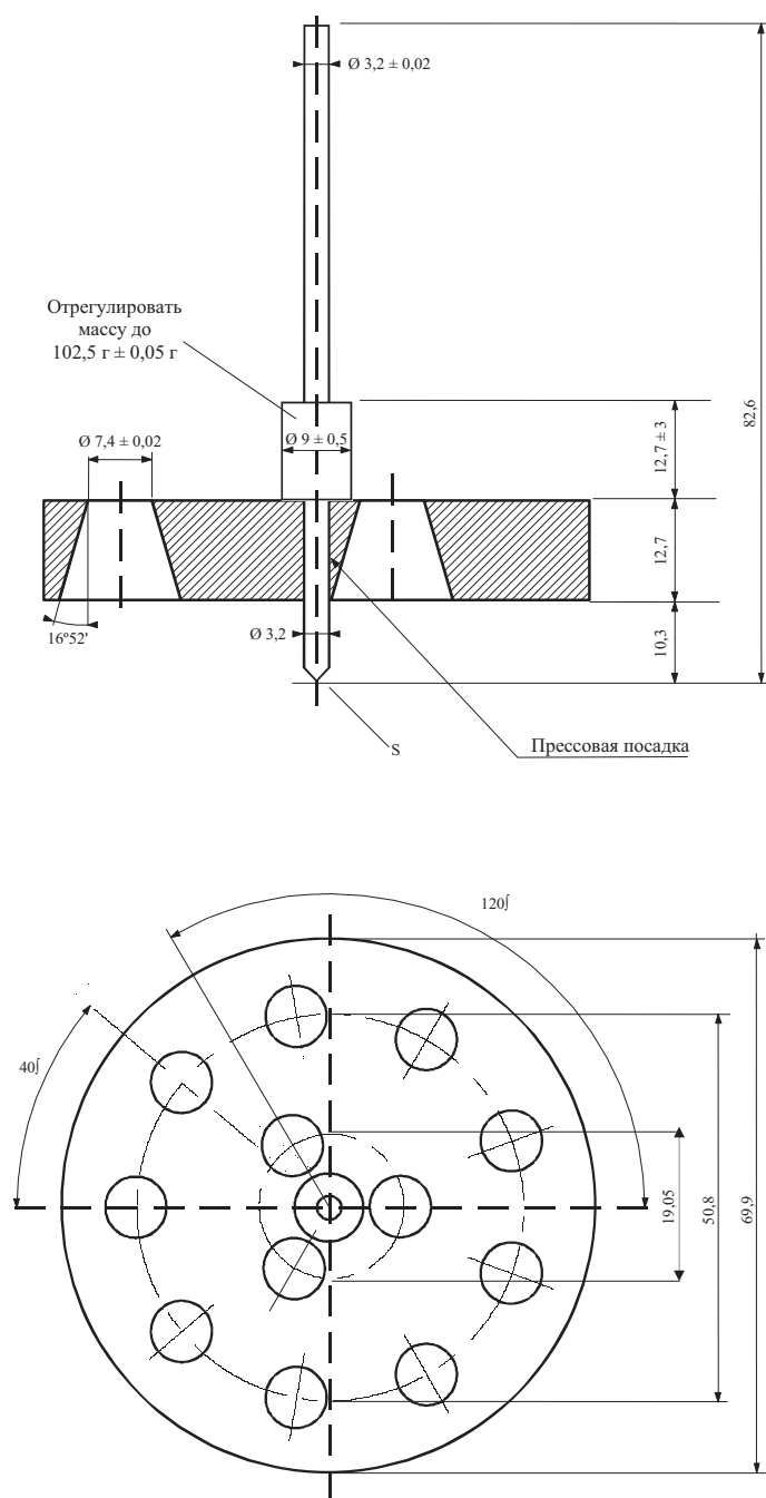
Рис. 1: Пенетрометр
